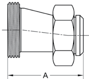
32TP (ECCENTRIC)
