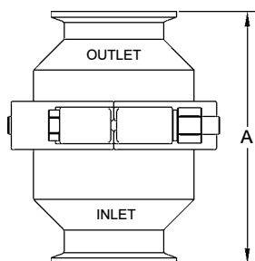
T45 / MC45
